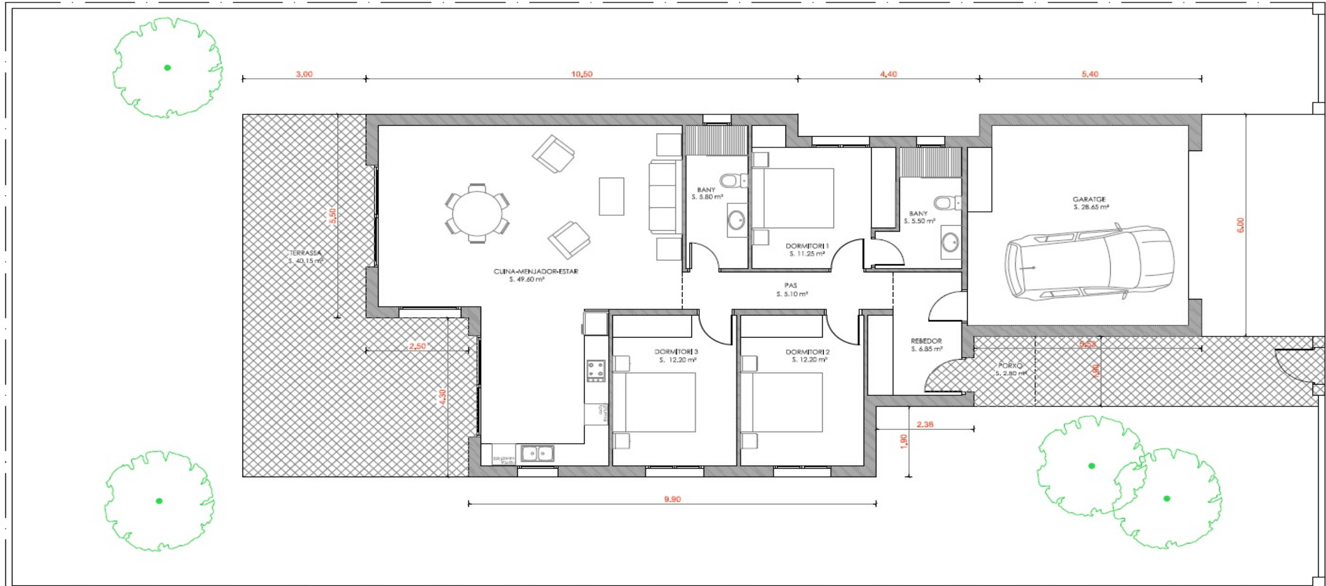
CASA 3 (VILAMACOLUM) PLANTA distribució, cotes i superfícies PROPOSTA 1
